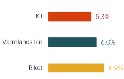
Figur 30: Långtidsarbetslöshet
