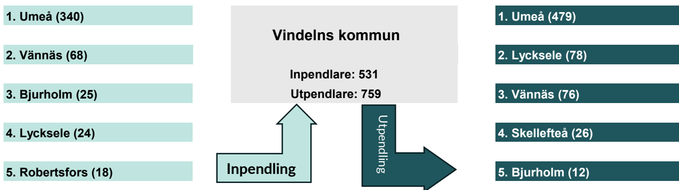
Figur 35: Pendling till och från Vindelns kommun 2024
