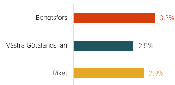
Figur 31: Ungdomsarbetslöshet
