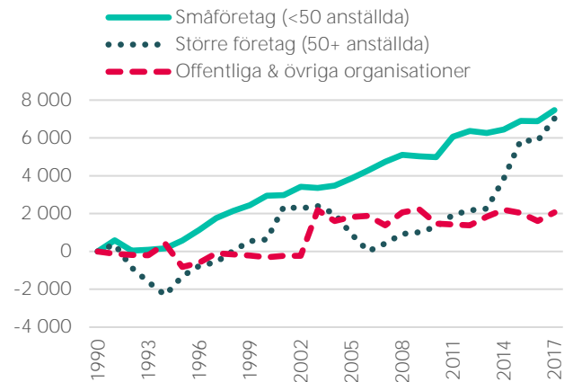
Utveckling antal jobb i Mölnads kommun 1990-2017
