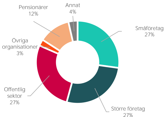
Andel av kommunala skatteintäkter per sektor, Mölnads kommun
