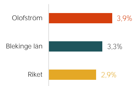
Figur 31: Ungdomsarbetslöshet
