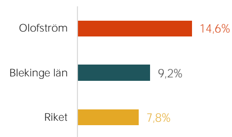
Figur 31: Ungdomsarbetslöshet
