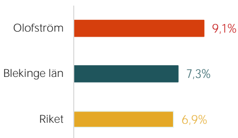
Figur 30: Långtidsarbetslöshet
