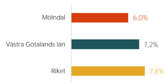
Figur 31: Ungdomsarbetslöshet
